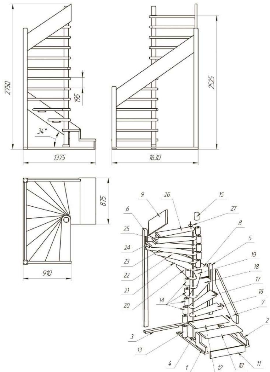
Рисунок 1. Лестница внутриквартирная ЛЕС-01.
